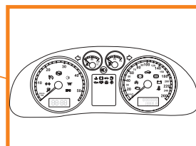
Schalttafeleinsatz mit Steuergerät für Wegfahrtsicherung und Diagnose-Interface (Gateway)
