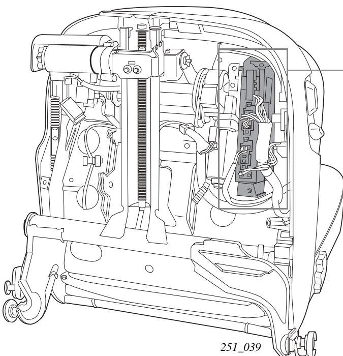
Steuergerät für Sitz- und Spiegelverstellung J394
