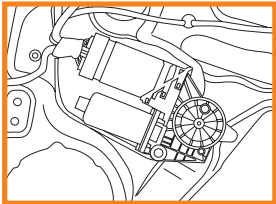
Fensterhebermotor mit integriertem Türsteuergerät
