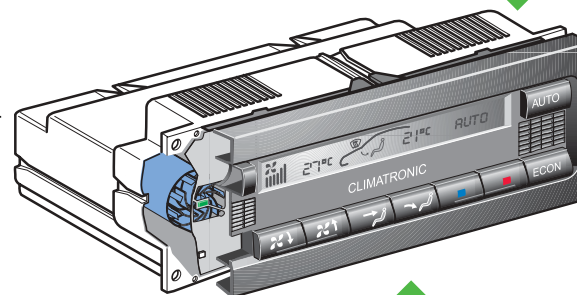
Climatronic-Steuergerät (hinter der Bedieneinheit)
