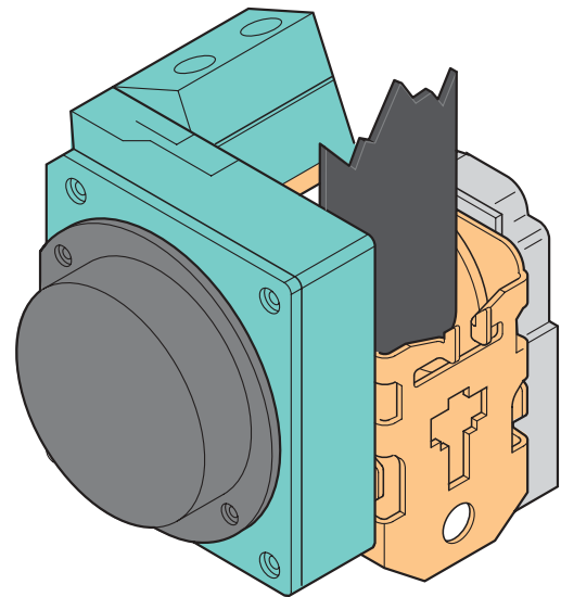
Wankelgurtstraffer
