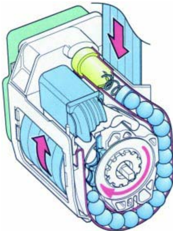
Kugelgurtstraffer
