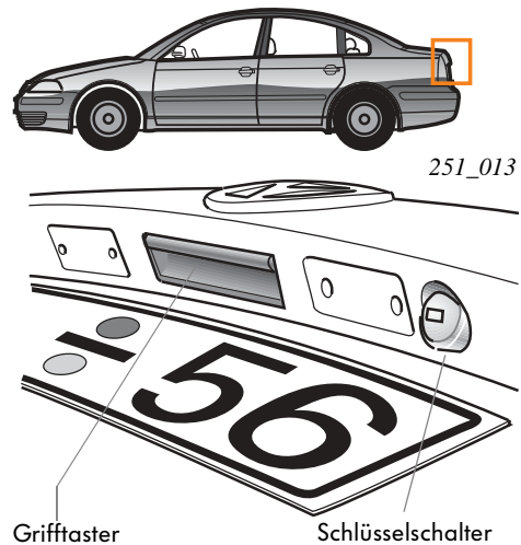
Schließkonzept Heckdeckel
