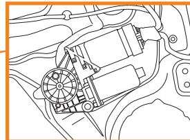
Fensterhebemotor mit integriertem Türsteuergerät
